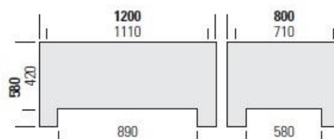
DIMENSIONES (mm):
