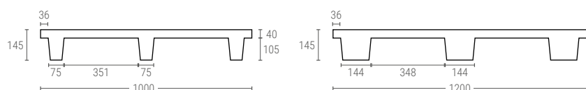
Innenmaße (mm)
